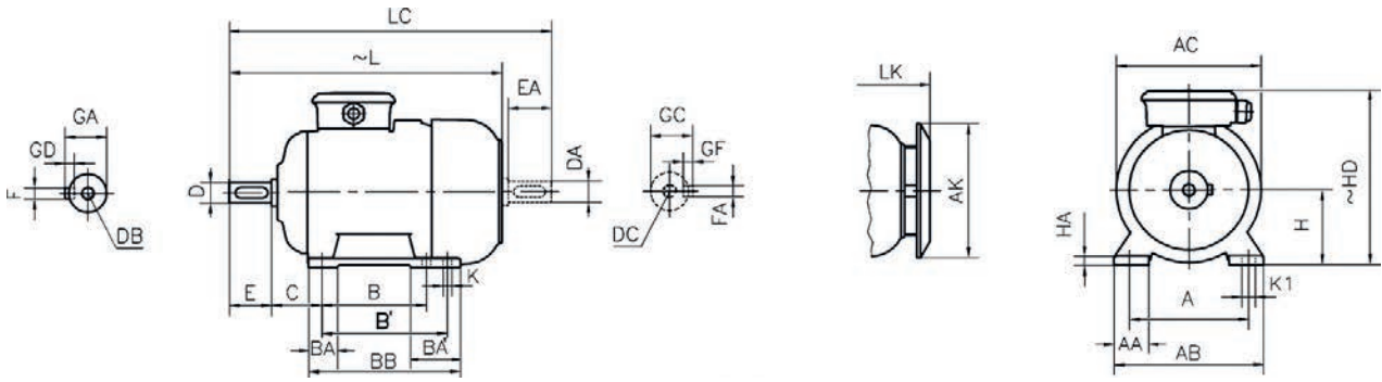
Ayaklı motor boyutları: B3, B6, B7, B8, B15, V5, V6 yapı biçimlerinde
