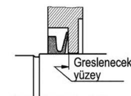
LASTİK TOZ CONTASI V-RING
