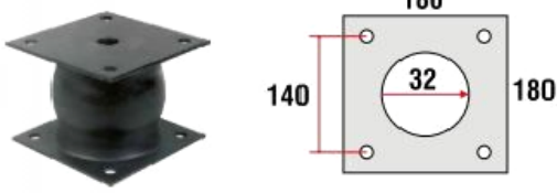
180'LİK ELEK TAKOZU / 180 Ø BUFFERS
